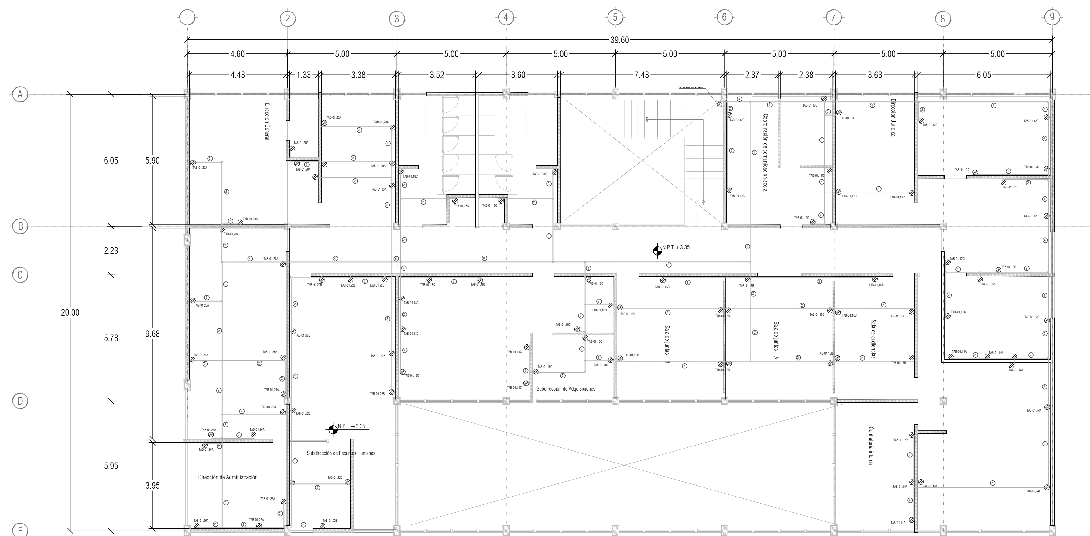
PLANTA ALTA
