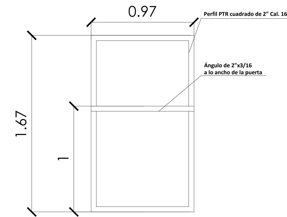
Detalle de puerta para nicho de medición
